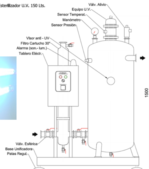
Equipo Esterilizador U.V. 150 Lts.
